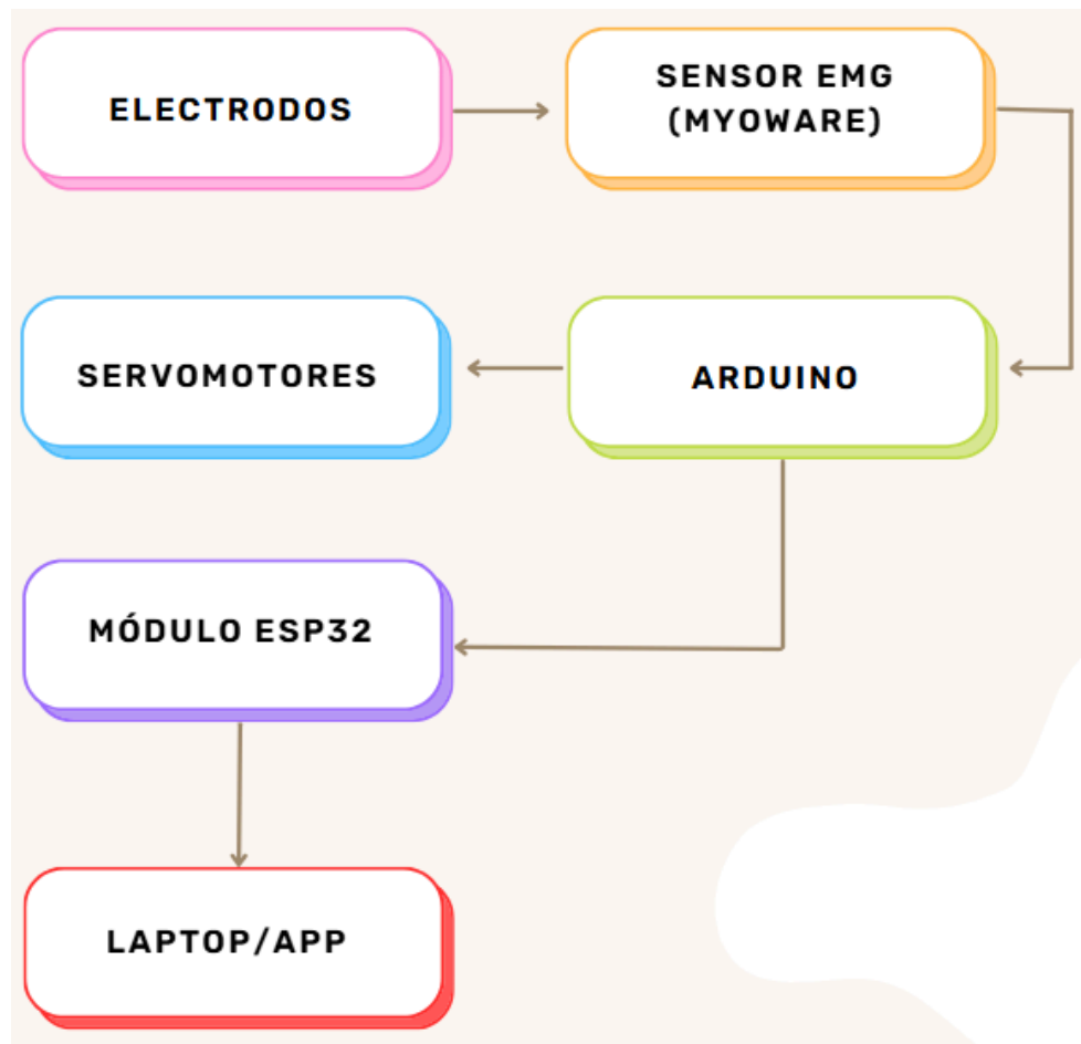
Figura 5: Esquema simple de conexión elaborada por nosotros
